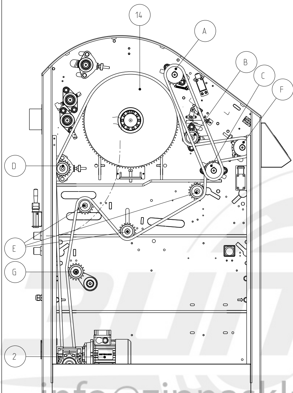
DETTAGLIO E
