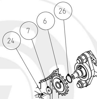
DETTAGLIO B
