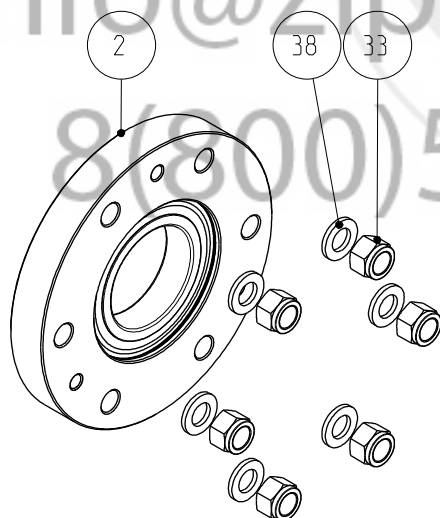
DETTAGLIO C
