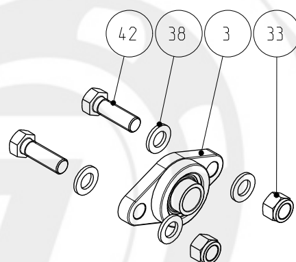
DETTAGLIO B
