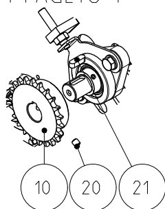
DETTAGLIO F
