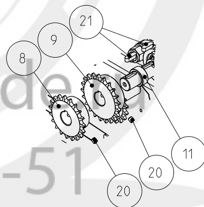
DETTAGLIO G
