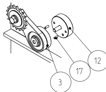
DETTAGLIO G
