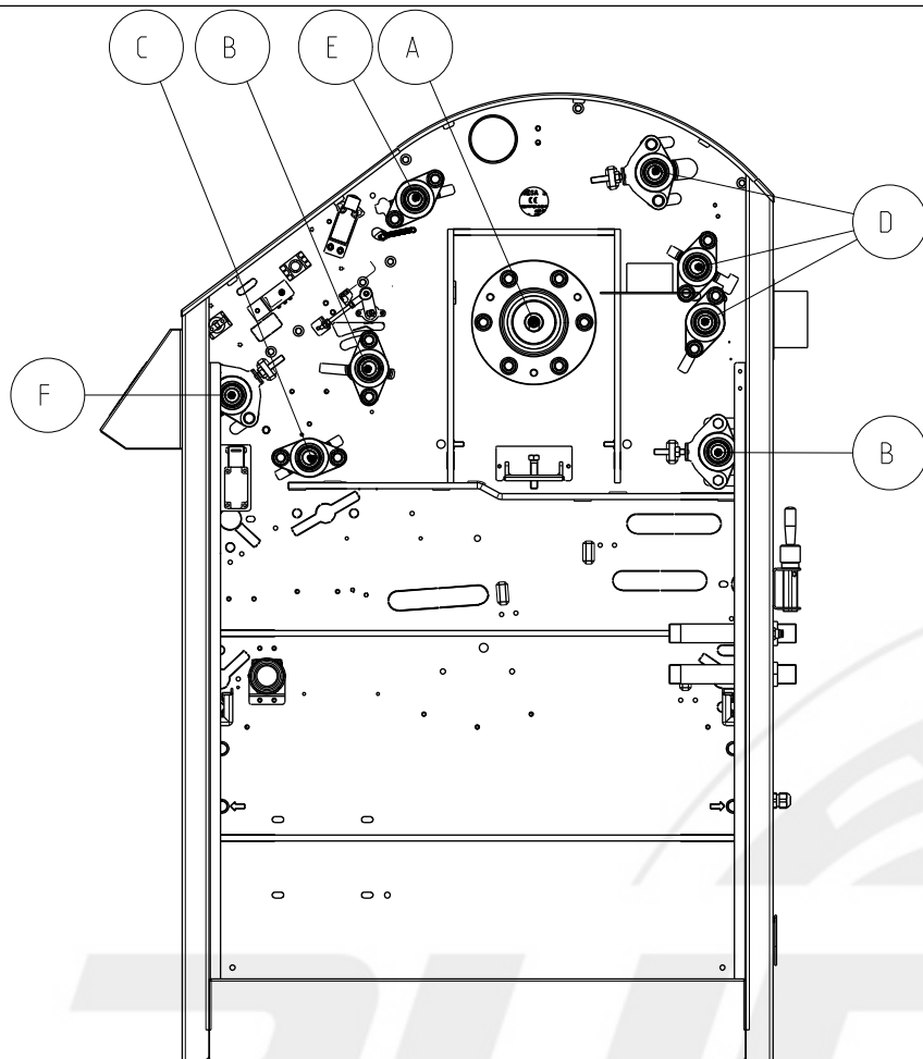
DETTAGLIO F
