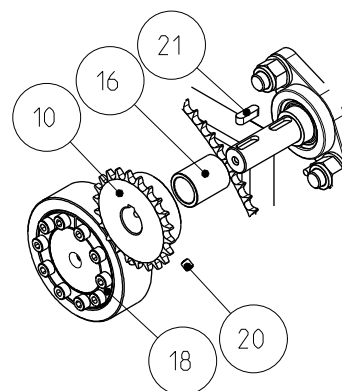
DETTAGLIO B
