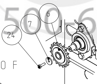
DETTAGLIO D
